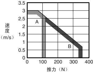
(2) SGTMF4B-036型
