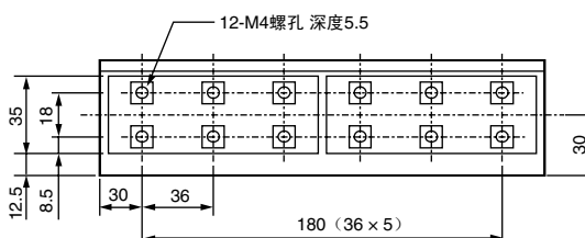
② SGLFW-35□230A□
