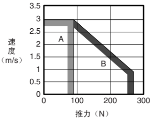
(1) SGTMF4A-027型
