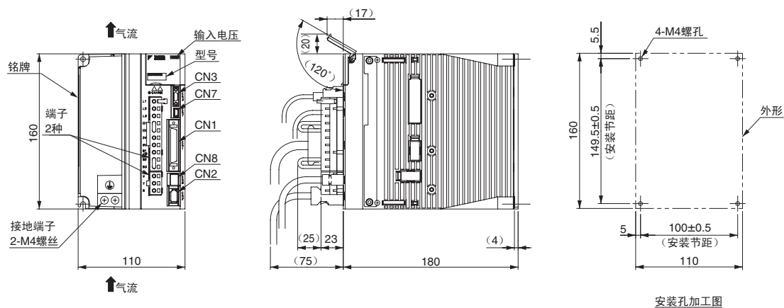
安装孔加工图
