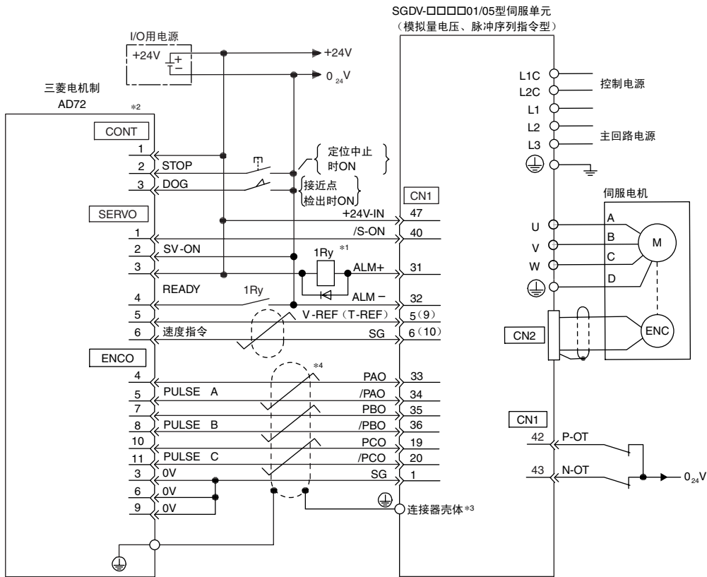
与三菱电机制定位装置AD72的连接示例（速度控制）
