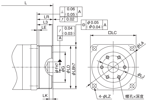
● 法兰输出详图
