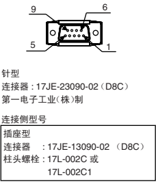
霍尔传感器用连接器规格
