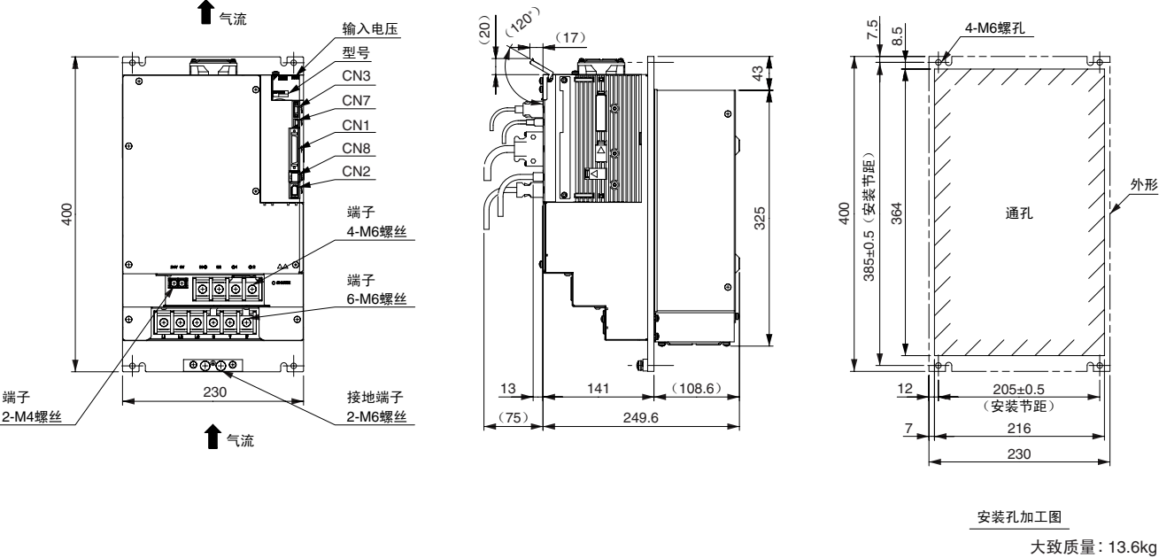
(15) 三相 AC 400V SGD V-280D0□A001、-370D0□A001 (通风管道安装型)
