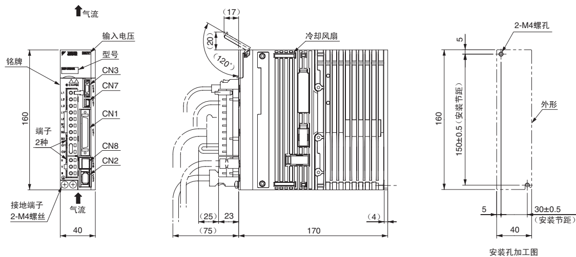
(5) 三相 AC200V SGD-3R8A0□A、-5R5A0□A、-7R6A0□A
