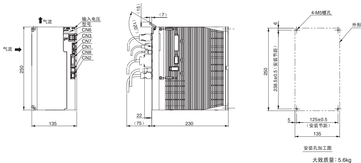
(13) 三相AC400V SGD-170D1□A
