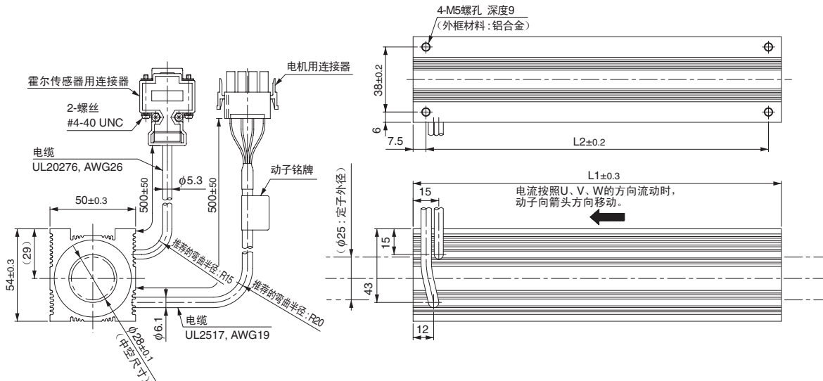
霍尔传感器用连接器规格
