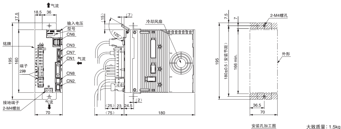
(6) 三相 AC200V SGD V-120A1□A001
