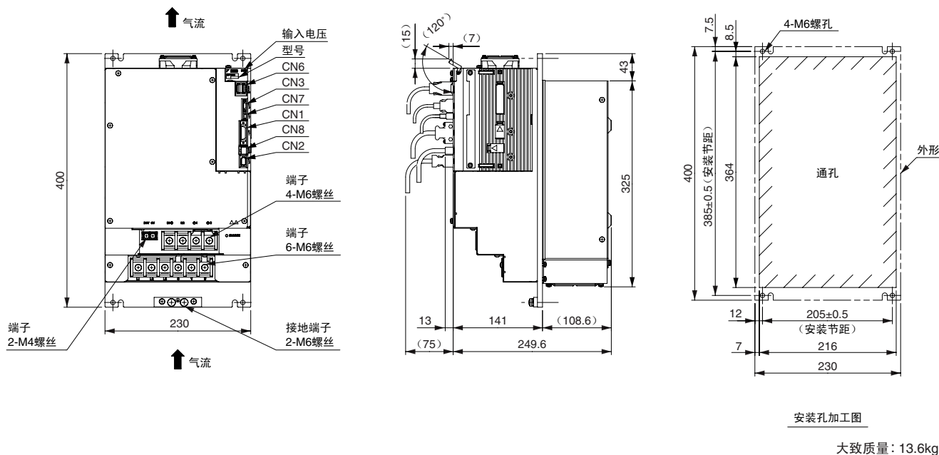
(15) 三相 AC 400V SGD V-280D1□A001、-370D1□A001 (通风管道安装型)
