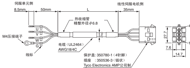
(1) 线性伺服电机主回路电缆 (JZSP-CLN11-□□-E 型)
