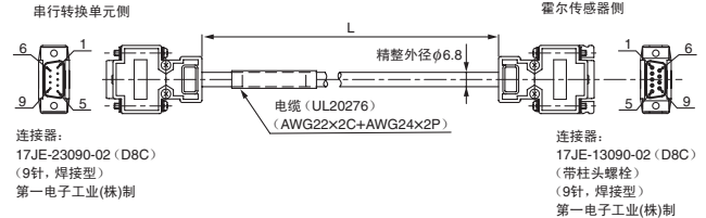
(4) 霍尔传感器连接电缆 (JZSP-CLL10-□□-E 型)
