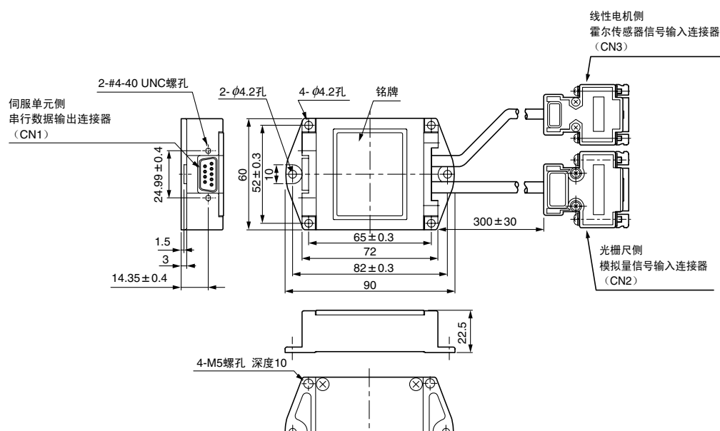
CN1
