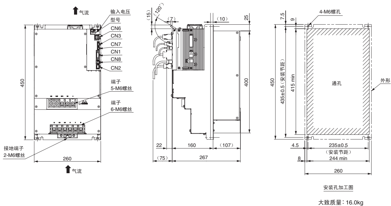
(10) 三相AC200V SGDⅤ-580A1□A001、-780A1□A001 (通风管道安装型)
