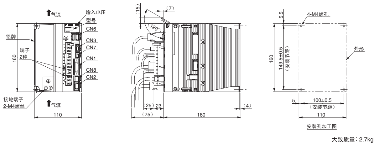
(12) 三相AC400V SGD-8R4D1□A、-120D1□A
