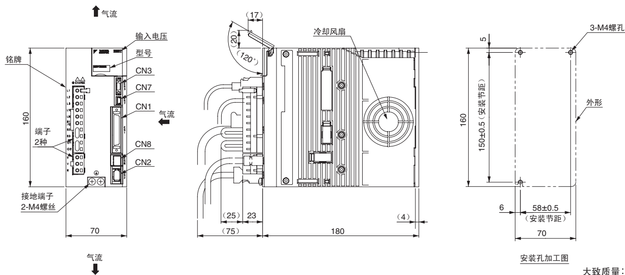
(6) 三相 AC 200V SGD-120A0□A
