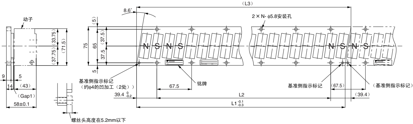
安装部详图
