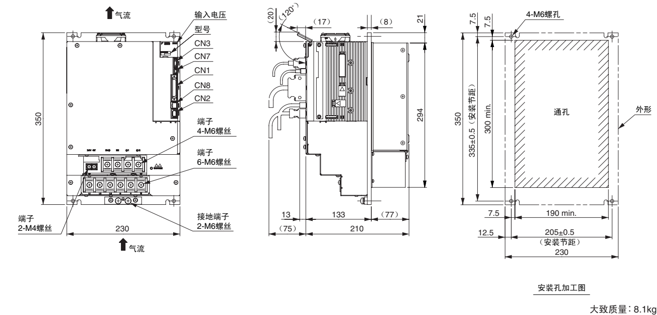
(14) 三相 AC 400V SGD V-210D0□A001、-260D0□A001 (通风管道安装型)
