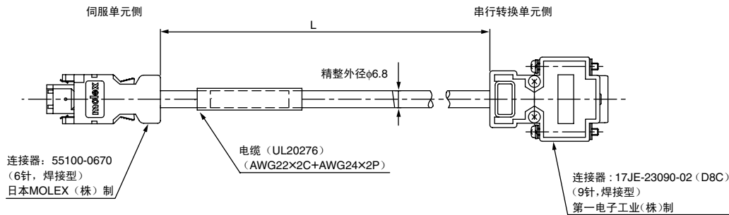
(6) 串行转换单元连接电缆 (JZSP-CLP70-□□-E 型)
