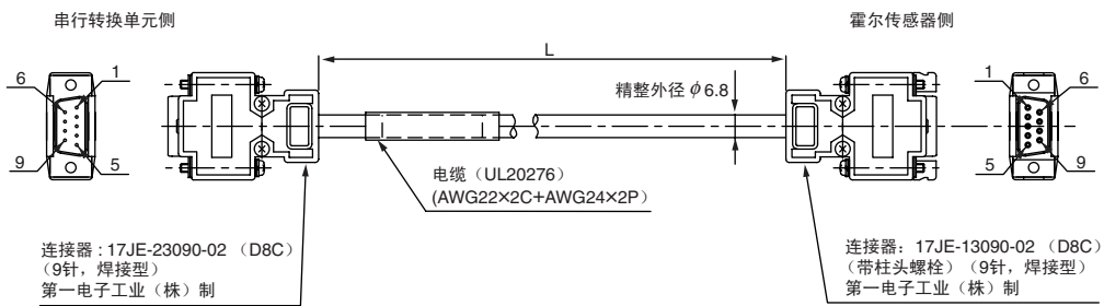
(7) 霍尔传感器连接电缆 (JZSP-CLL10-□□-E 型)
