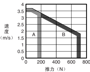
（2）SGTMF5B-072型
