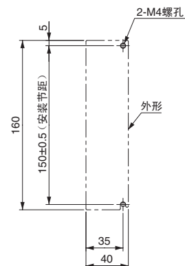
安装孔加工图
