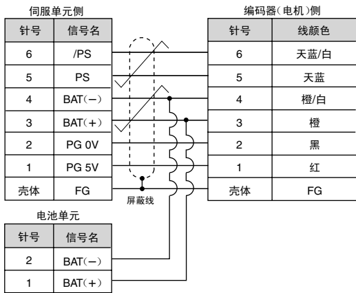
(3) 带电池单元的电缆接线规格
