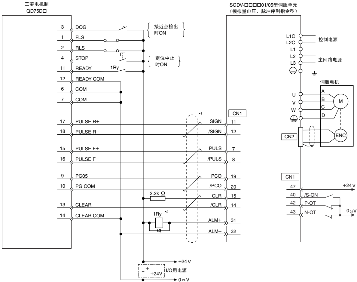
与三菱电机制定位装置 QD75D□ 的连接示例（位置控制）
