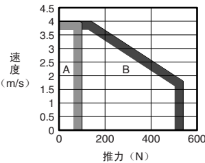
（1）SGTMF5A-054型
