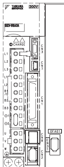
安装于模拟量、脉冲型伺服单元的正视图
