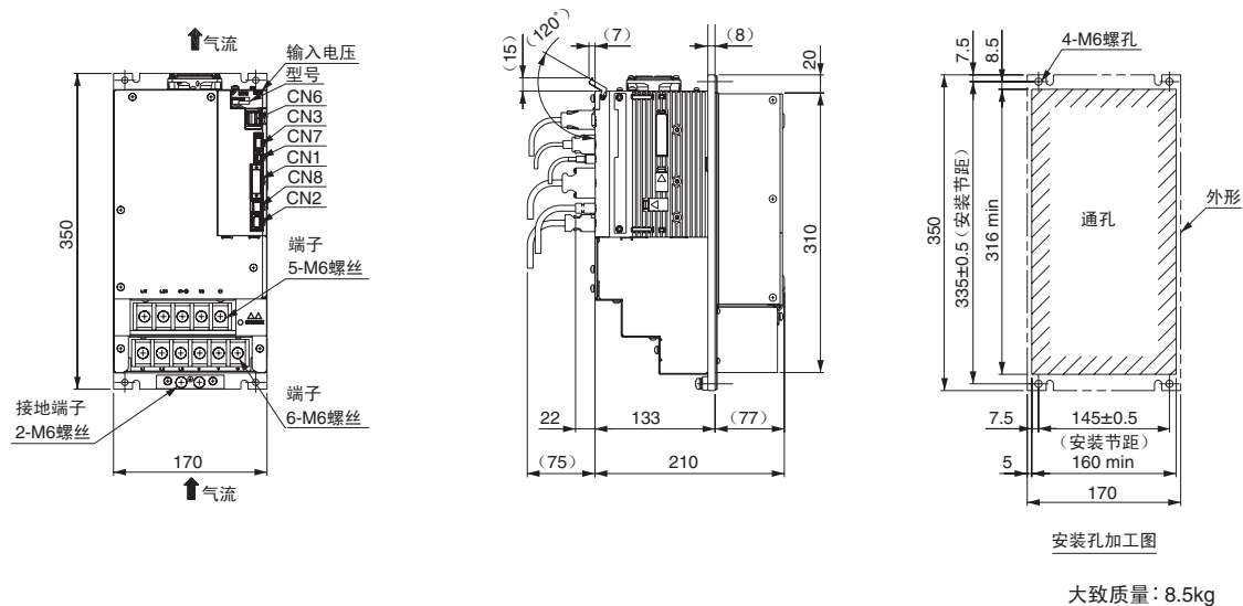
(9) 三相AC200V SGDⅤ-470A1□A001、-550A1□A001 (通风管道安装型)
