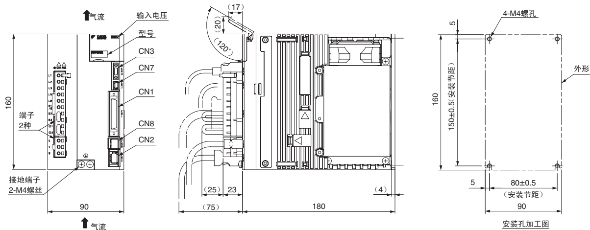
(6) 三相 AC 200V SGD-120A0□A
