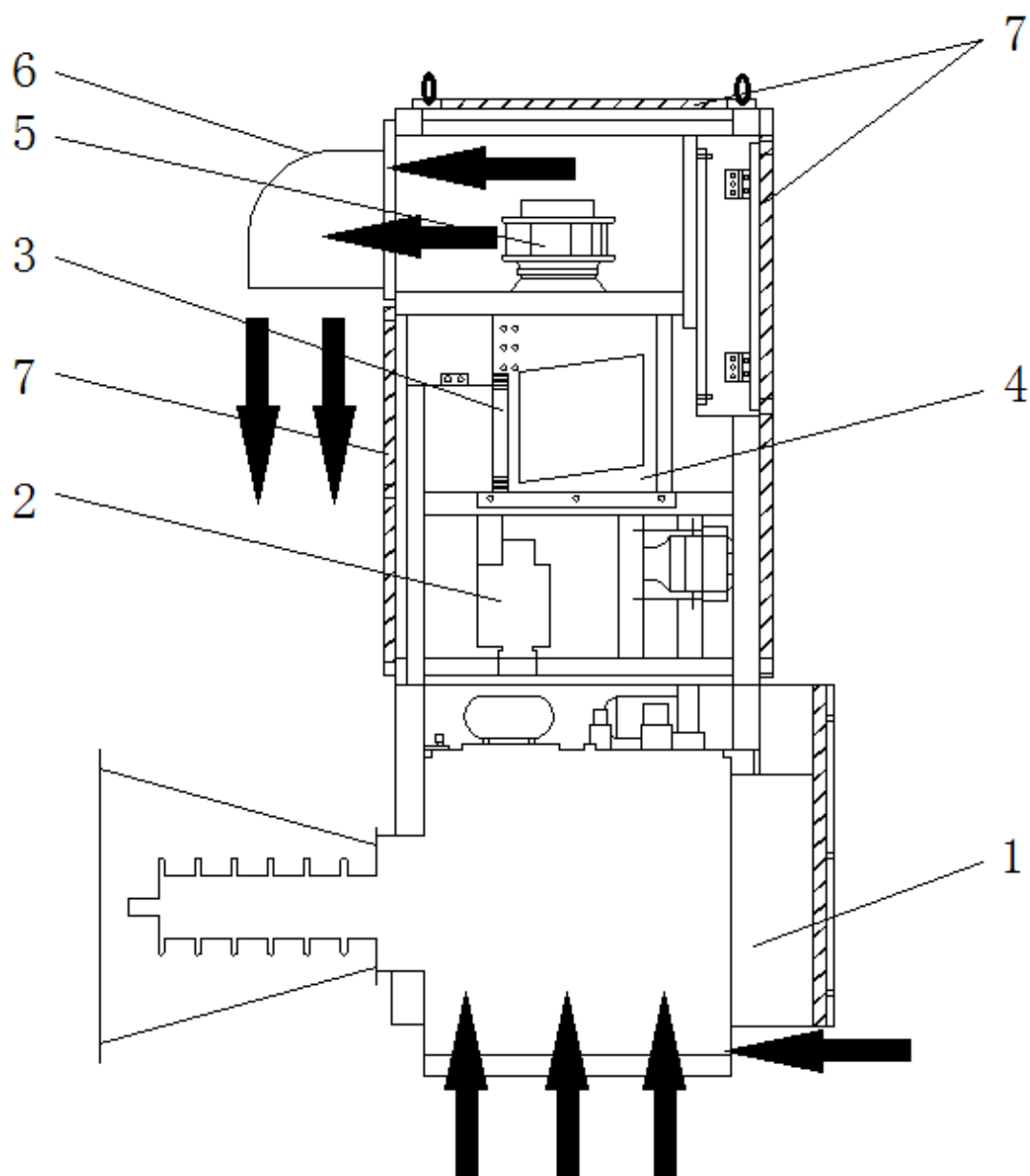
图 2 结构布局散热示意图
