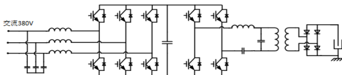
图1 主电路原理示意图
